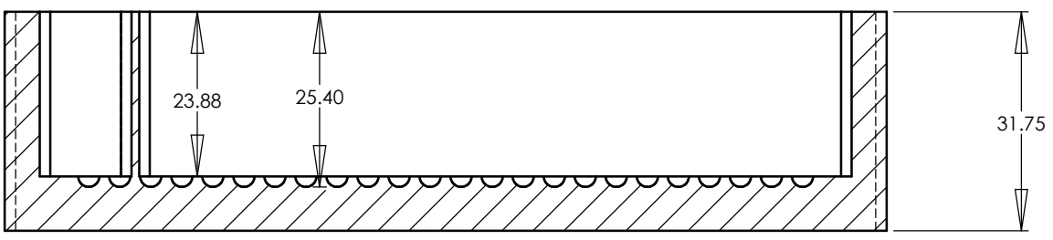
SECTION A-A SCALE 1 : 1
